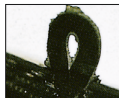
Coupe d'une cheville FLOW-SEAL placée dans un pneu Radial qui a été testé sur une distance de 81000 km
